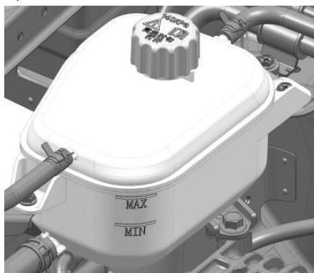
Расширительный бачок
